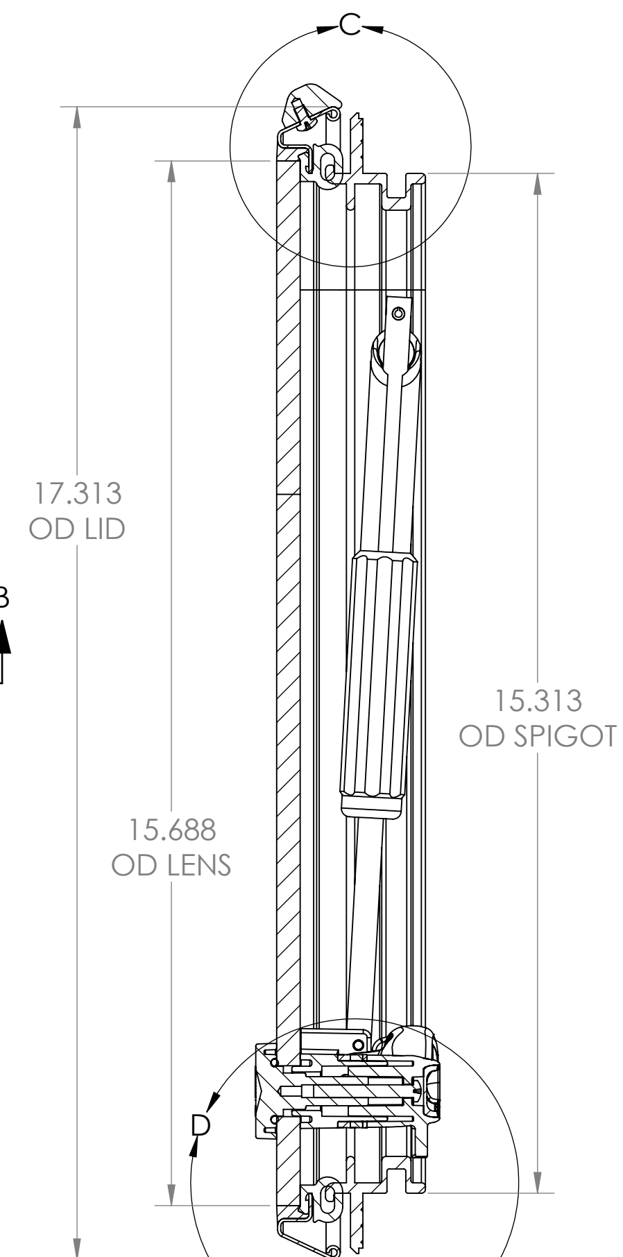
SECTION A-A
