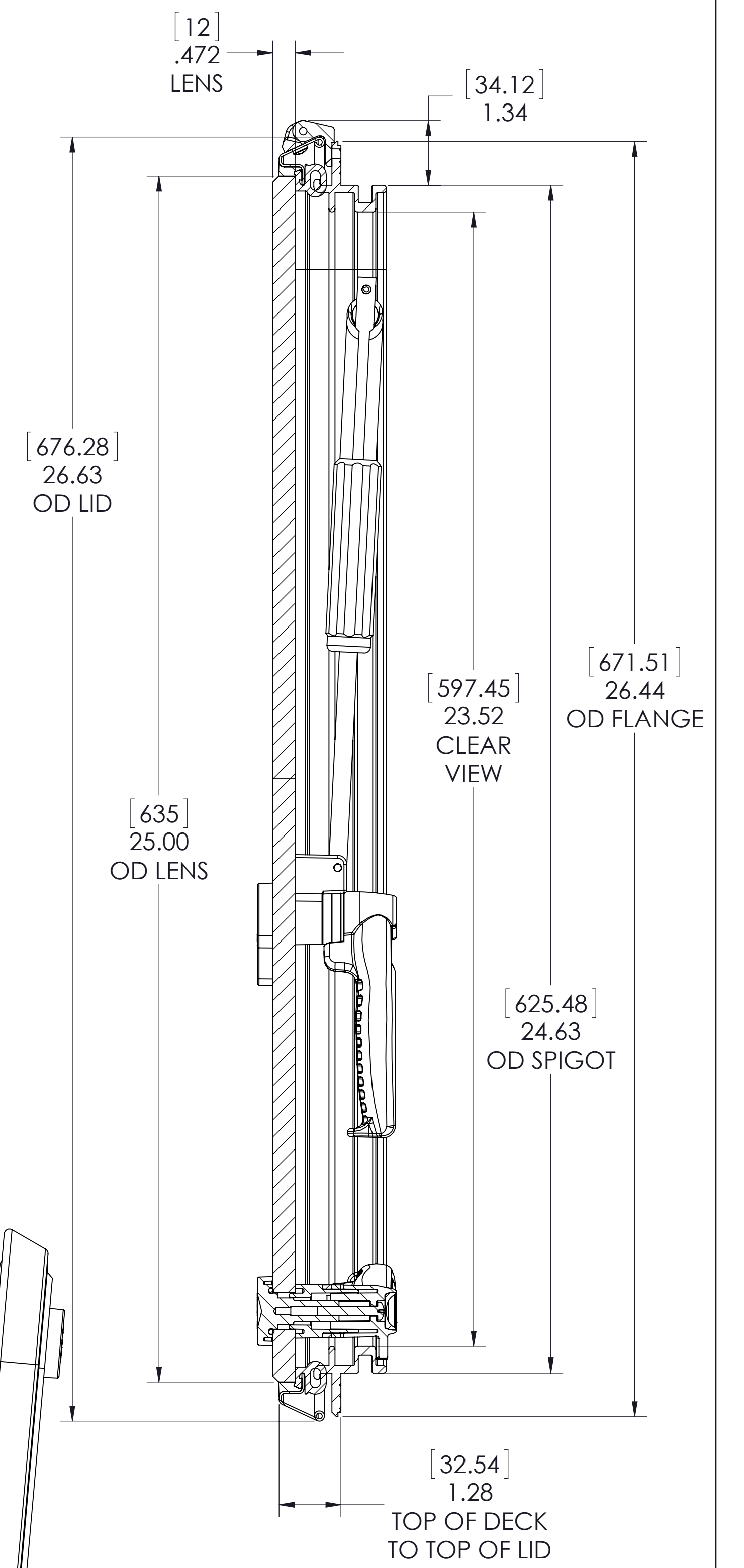
SECTION A-A
