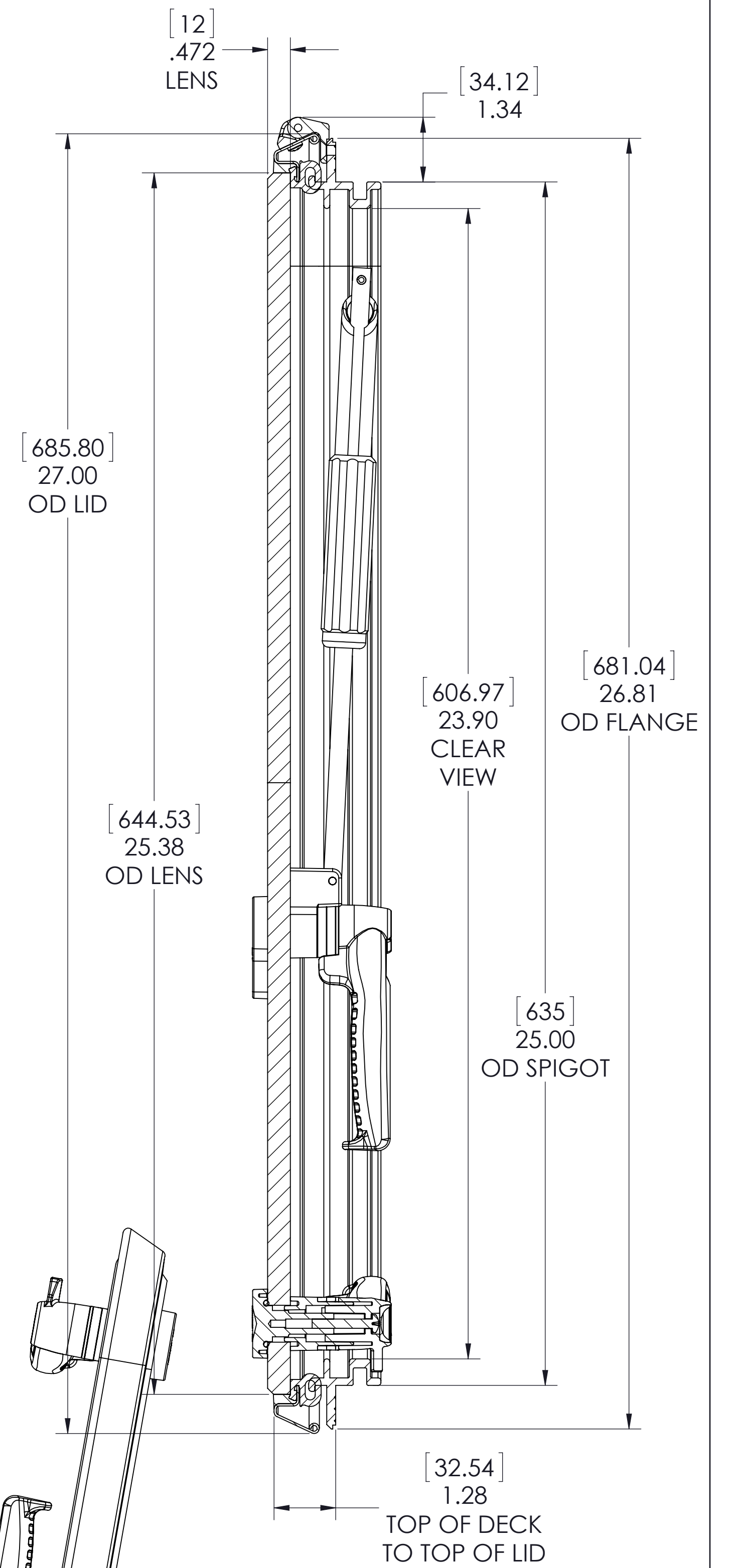
SECTION A-A
