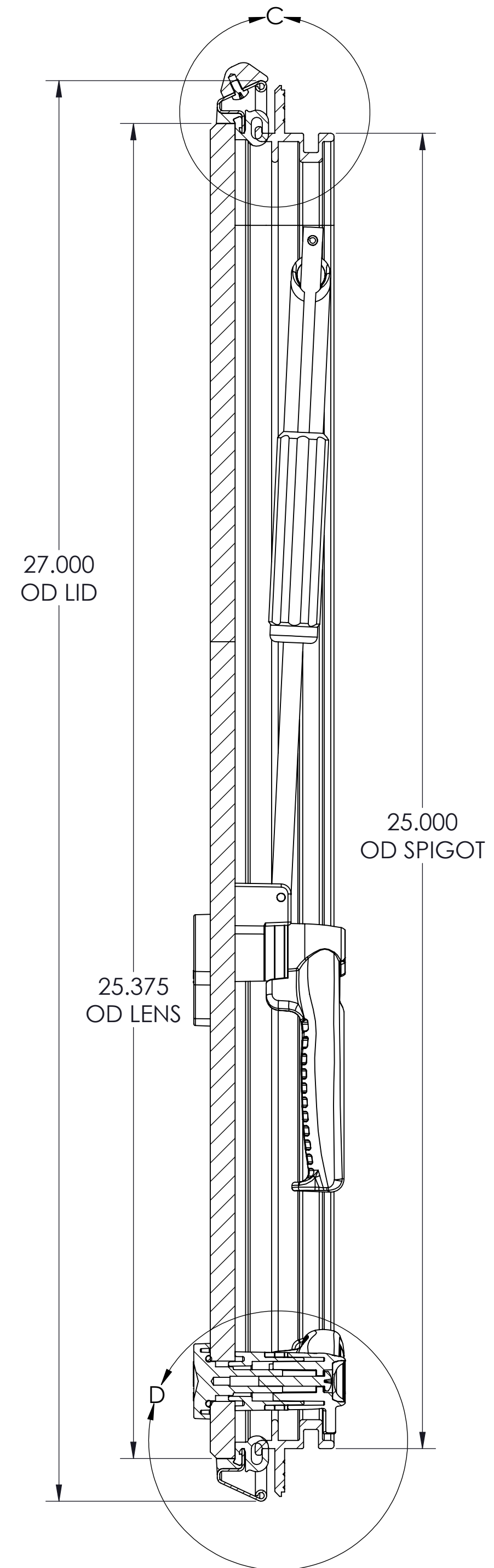
SECTION A-A
