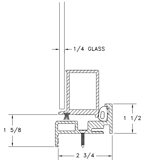
SECTION THRU DOOR PANEL
