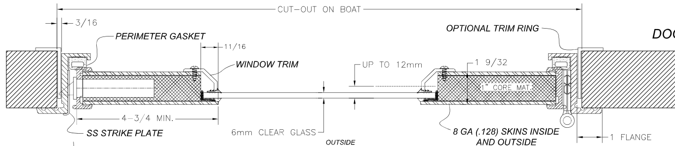
SECTION A-A
