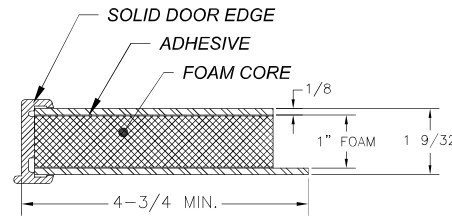
DOOR PANEL
