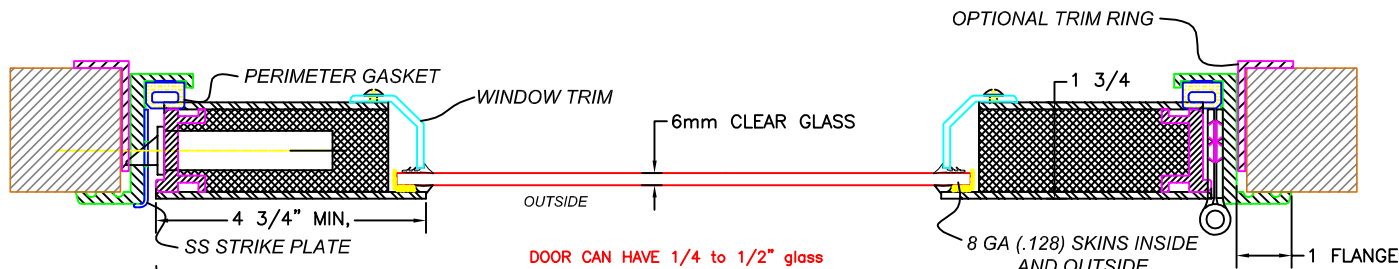
SECTION A-A
