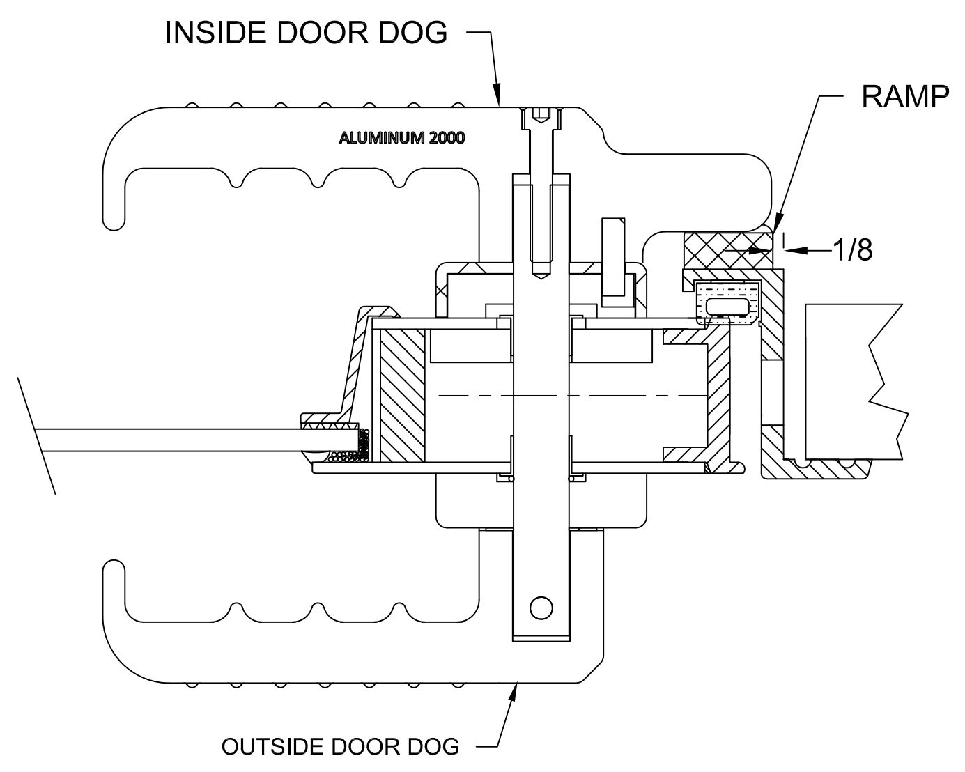
OPTIONAL DOOR DOG DT'L
